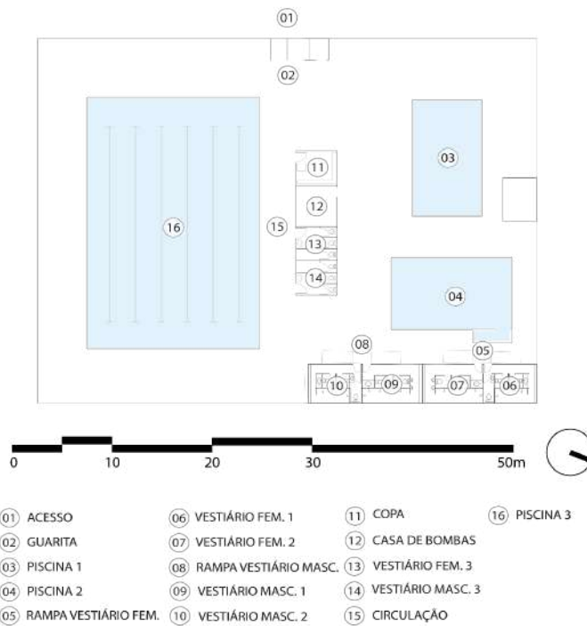
Figura 07: Planta baixa atualizada pelo Lacesse do Parque Aquático da UFPB.
