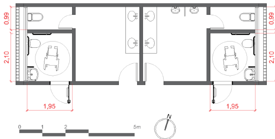
Figura 05: Proposição para WC's no térreo do CTH.
