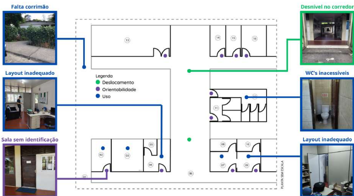
Figura 13: Mapa de análise do Bloco Administrativo.
