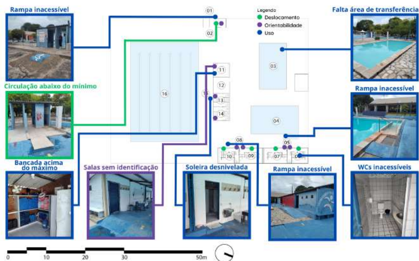
Figura 08: Mapa de análise do Parque Aquático.
